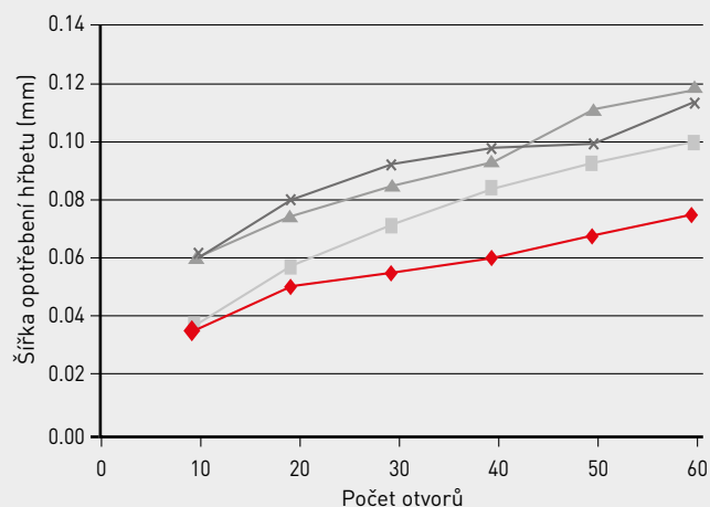
Šířka opotřebení hřbetu po vyvrtání 60 otvorů
